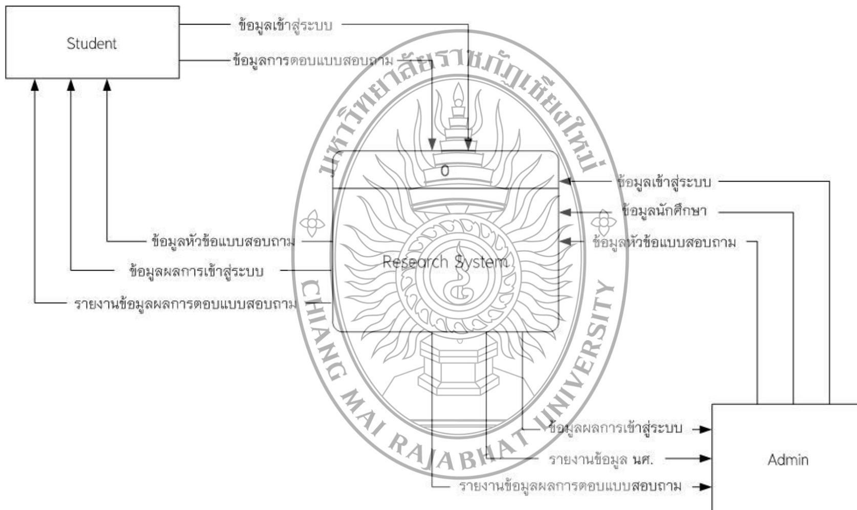
ภาพที่ 4.2 ภาพรวมของระบบ (Context Diagram)
